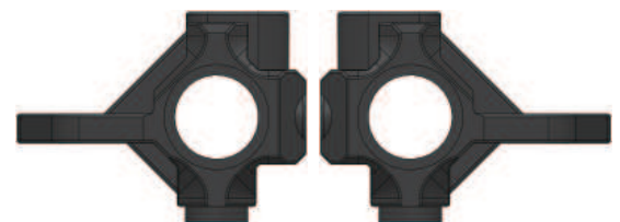
KPI Steering Block - L (1) / R (1) KPIステアリングブロック - L (1) / R (1)
